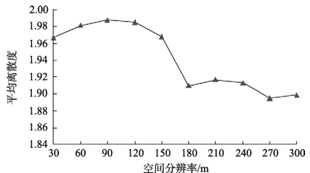
图10 TM影像上描述类别可分性的平均离散度随空间尺度变化图
