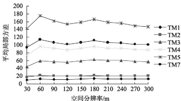
图8 TM影像上各个波段的平均局部方差随空间尺度变化图
