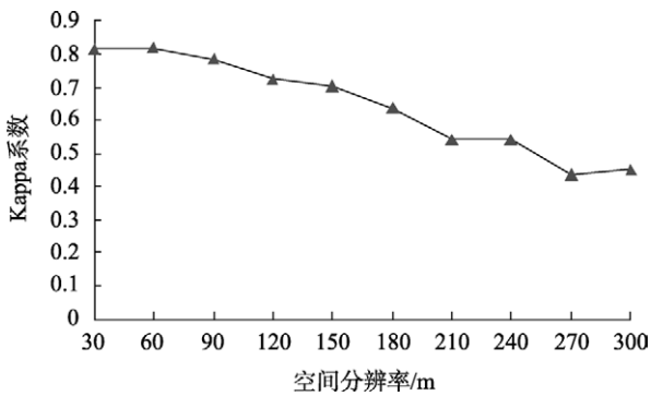
图7 TM影像上 Kappa 系数随空间尺度变化图
