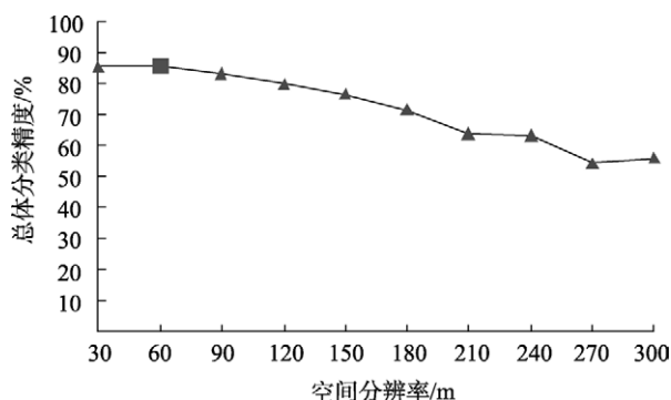
图 12 QuickBird 影像上总体分类精度随空间尺度变化图
